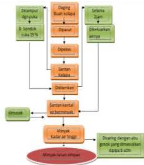
Gambar 3. Diagram Alir Pembuatan Minyak Tahan Simpan
